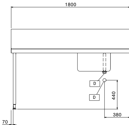
Zij aanzicht
